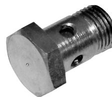
2788 16.290.106 Parafuso Oco 16 x 1,5 curto Monza e outros
