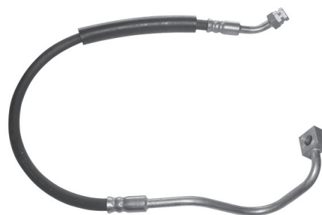
1104 2SH 607183-A F-4000 Lado Direito 93... 660 mm
