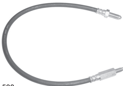
1604 5.954.603 Uno-S / CS / Premio / Fiorino / Elba ...87 - 380 mm
