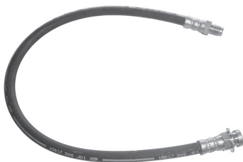
1527 RE 00328 Trafic - 383 mm / Trafic - 425 mm
